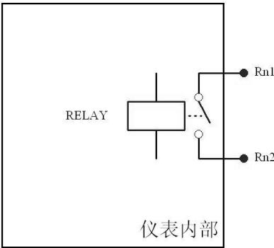
图 3.2 继电器输出接口电路示意图
