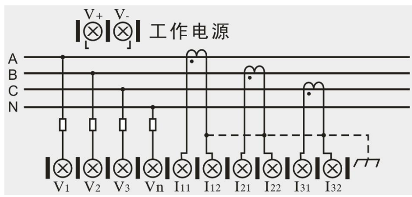
图 5.3 三相四线(无 PT)接线图
