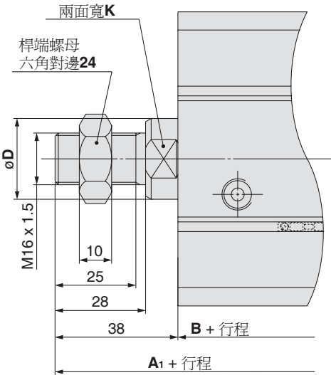
基本型氣缸
